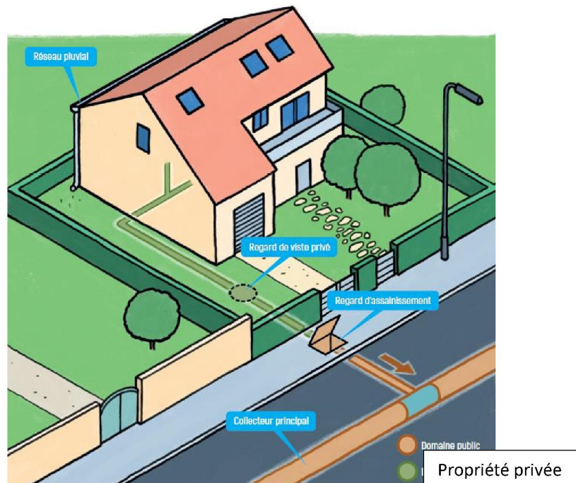
Figure 1 : situation de conformité avec le règlement de service
