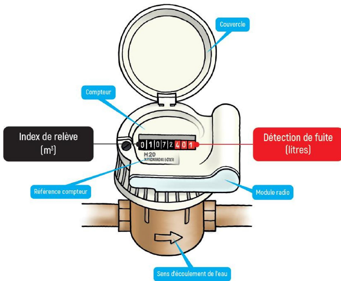
Figure 1 : Vue éclatée d'un compteur radio-relevé
