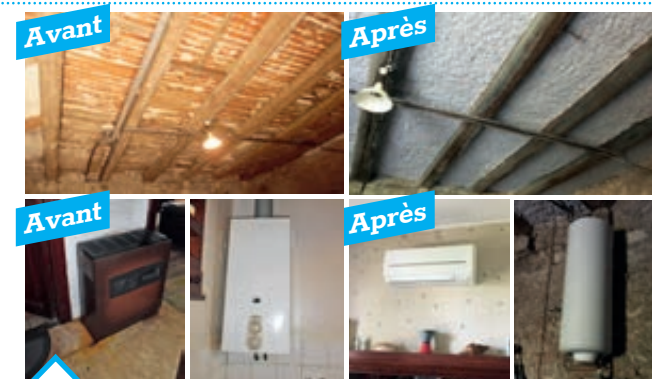
Travaux de rénovation énergétique d'une maison vigneronne à Campagnan (cf. témoignage). Les aides de Rénovissime ont notamment permis la réfection et l'isolation de la toiture, le changement du système de chauffage (le poêle à mazout a été remplacé par une pompe à chaleur) et l'installation d'un cumulus électrique.
