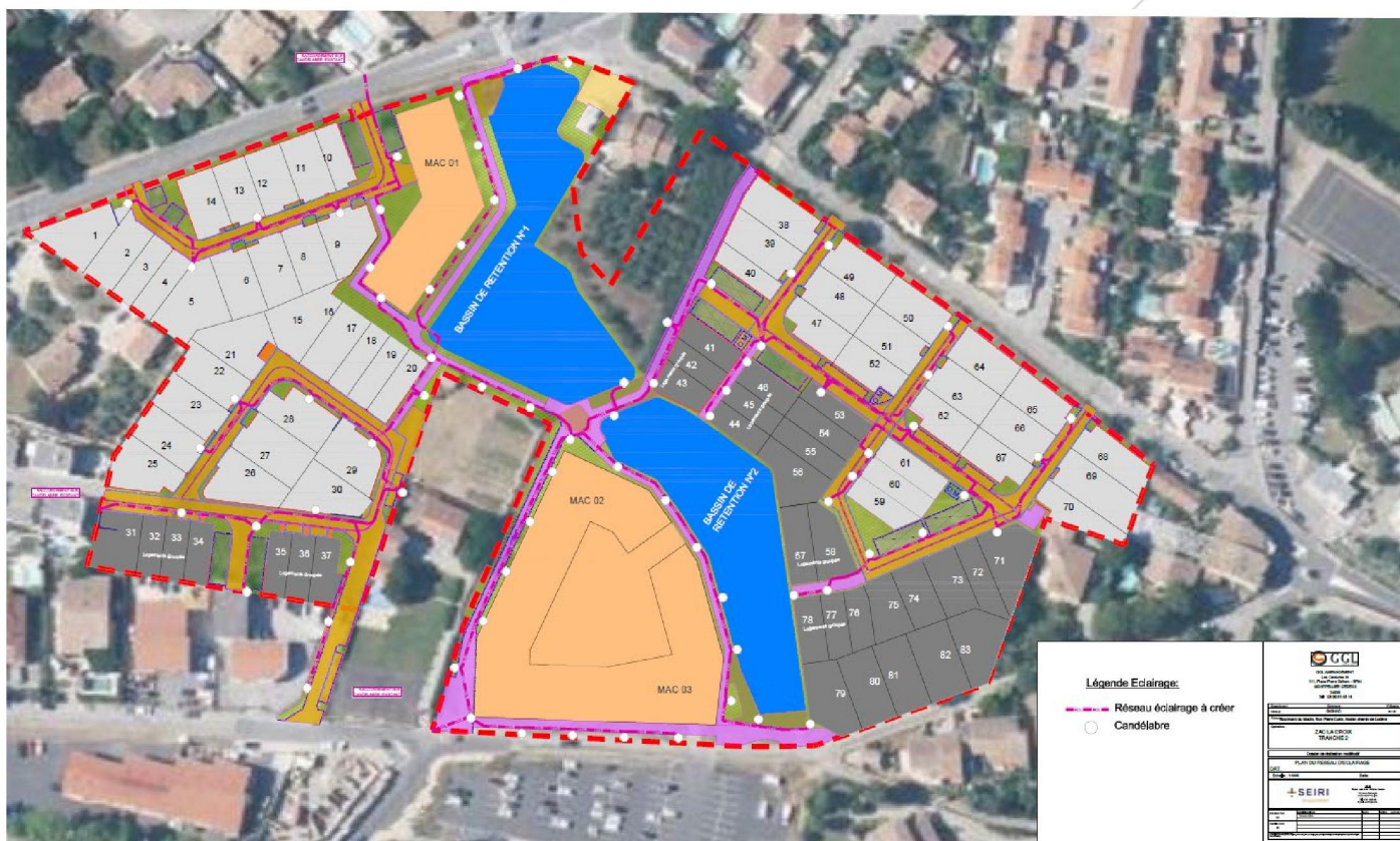
Plan indicatif de l'éclairage public
