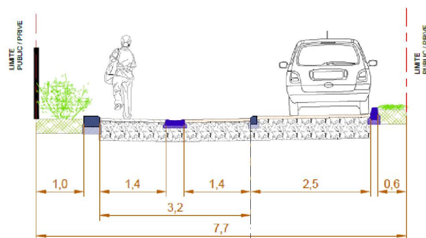
Chaussé à sens unique | Stationnement
